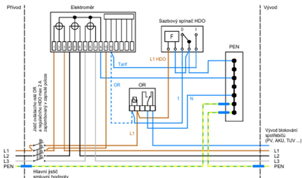
Obrázek 6 - Schéma úpravy zapojení ER s dvoutarifní sazbou pro 3fázové měření typu C a HDO, připravená pro budoucí Sdílení a montáž elektroměru typu B
