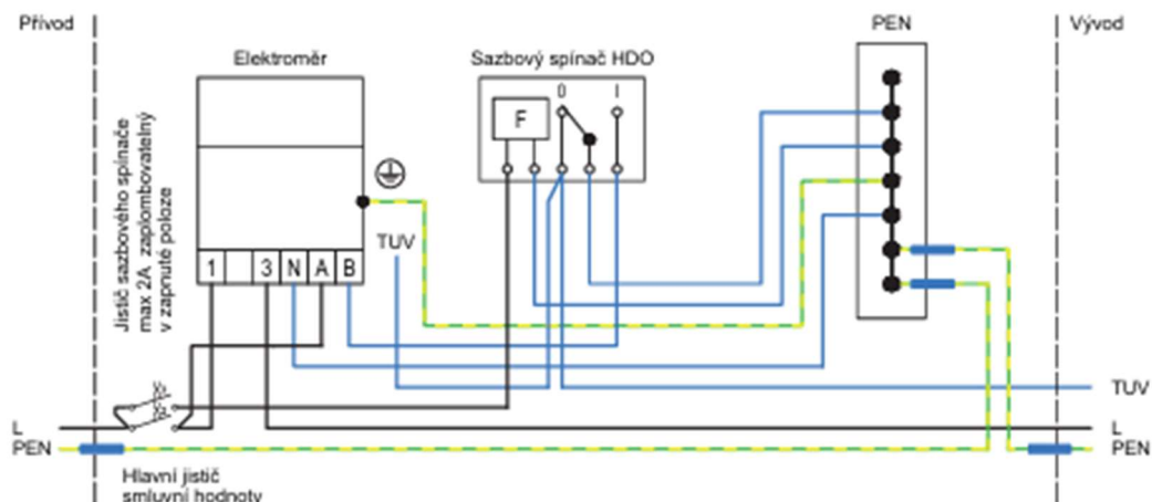
Obrázek 7 – Schéma úpravy zapojení ER s dvoutarifní sazbou pro 1fázové měření typu C a HDO, připravená pro budoucí Sdílení a montáž elektroměru typu B
