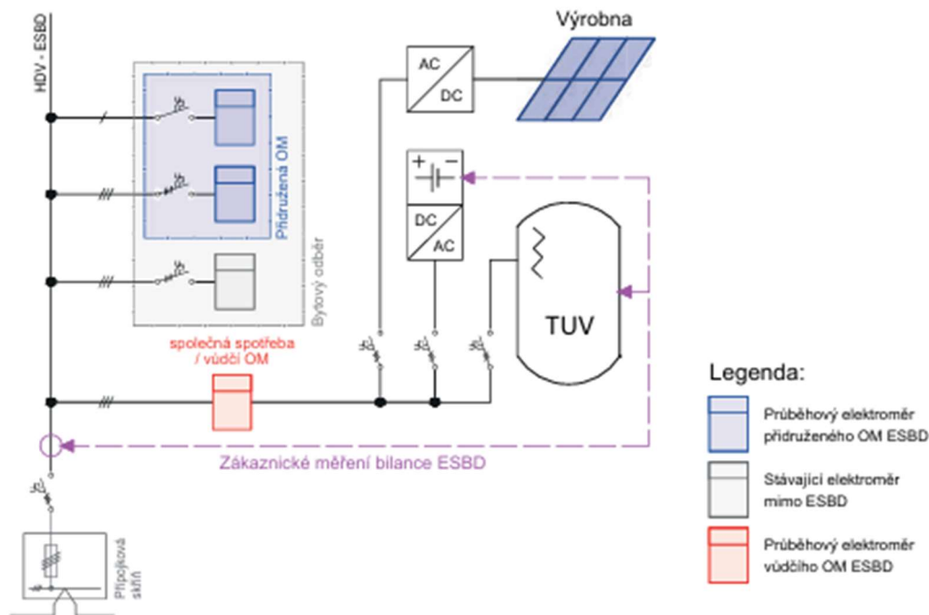
Obrázek 9 - Zapojení instalace pro ESBD s vůdčím OM, přidruženými i nepřidruženými OM
