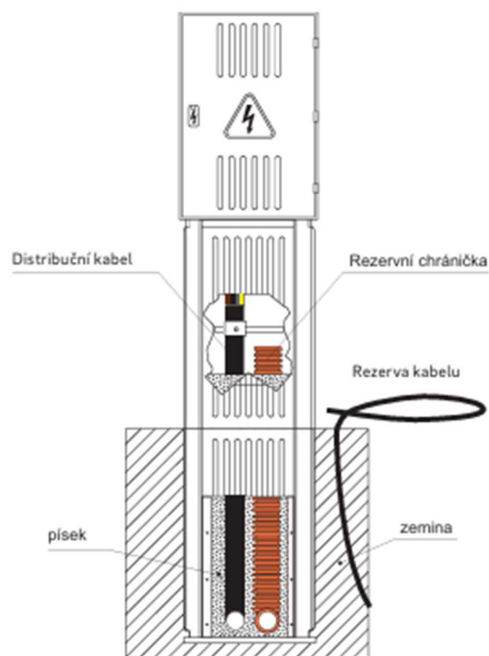
Obrázek 2 - Přípojková skříň v pilíři se založenu chráničkou
